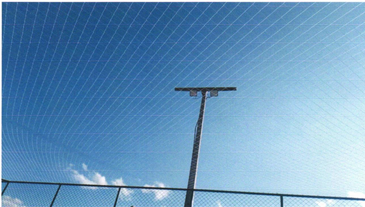
Foto 05 - Refletor Slim LED 200W de potência, branco Frio, 6500k, Autovolt, marca G-light ou simila
